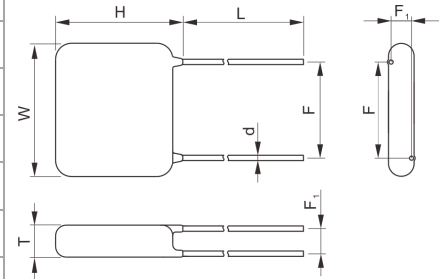
直型引线 Straight Lead
