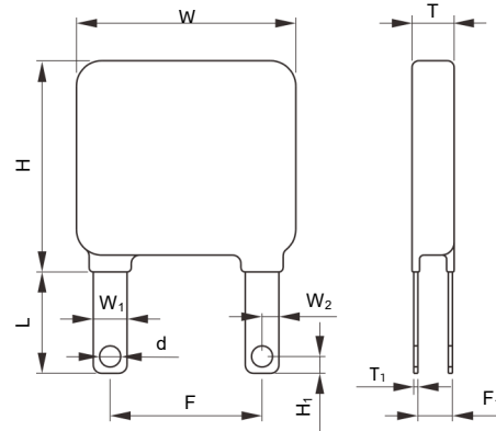
直带型端子 Straight Strap Terminals
