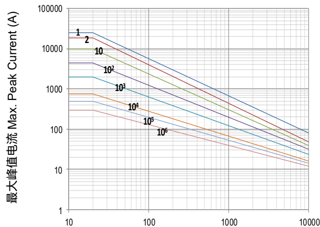
脉冲持续时间 Impulse Duration (μs) SFV25S820K to SFV25S122K
