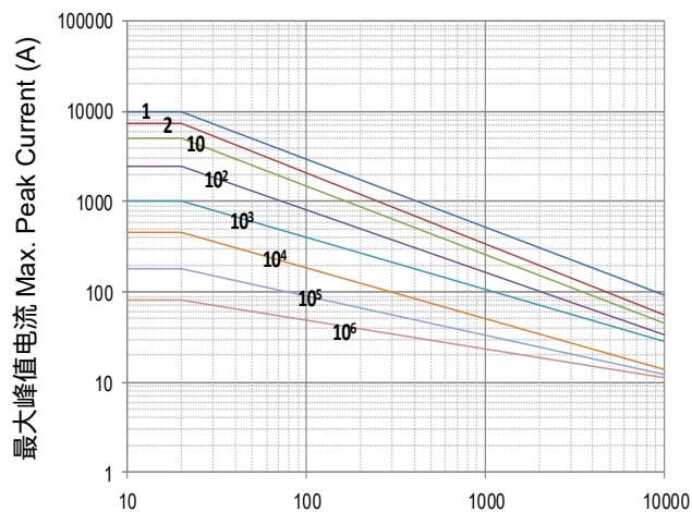
脉冲持续时间 Impulse Duration (μs) SFV25S220K to SFV25S680K
